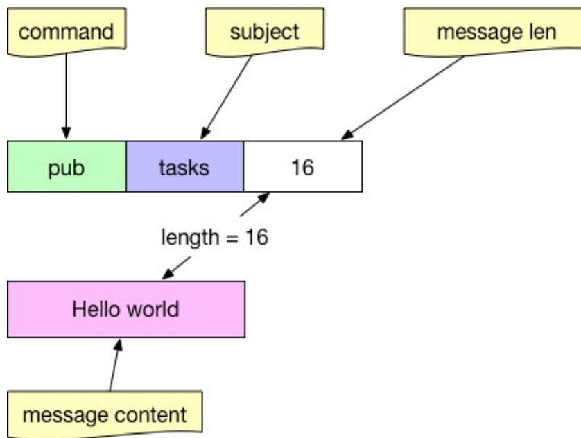
Pub trong giao thức NATS
