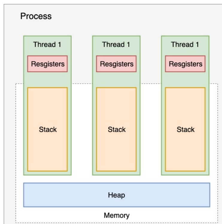
Mô hình xử lý song song
