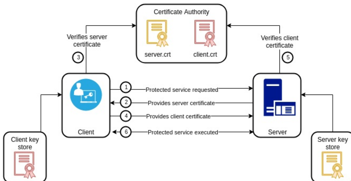
Xác thực bằng chứng chỉ
