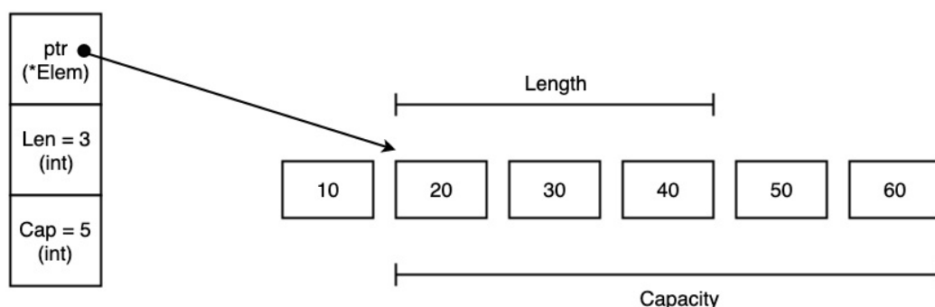
Cấu trúc Slice
