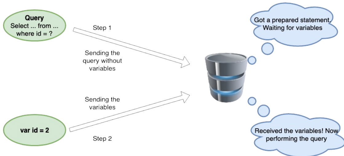
Minh hoạ cơ chế Prepare statement
