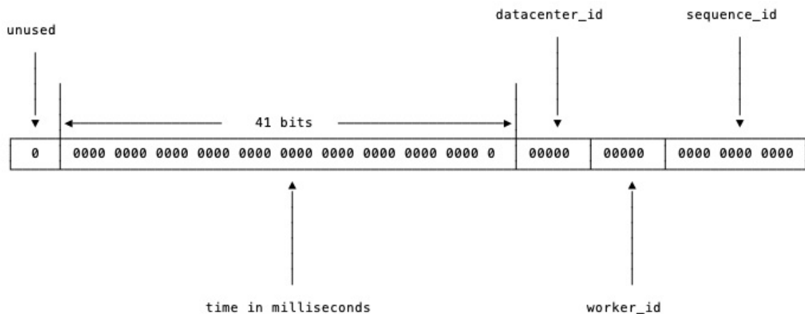
Phân phối Bit trong snowflake
