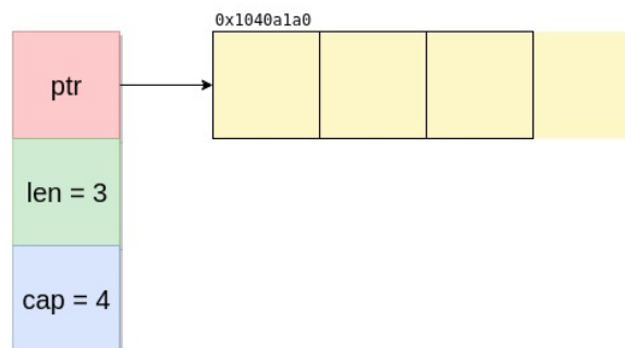
Mình hoạ slice
