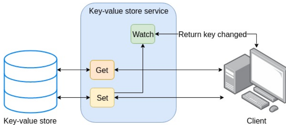
Mô hình sử dụng hàm Watch
