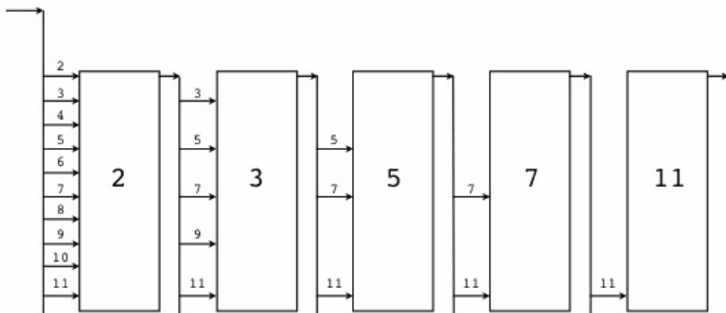
Sàng số nguyên tố
