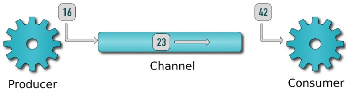
Mô hình Producer - Consumer
