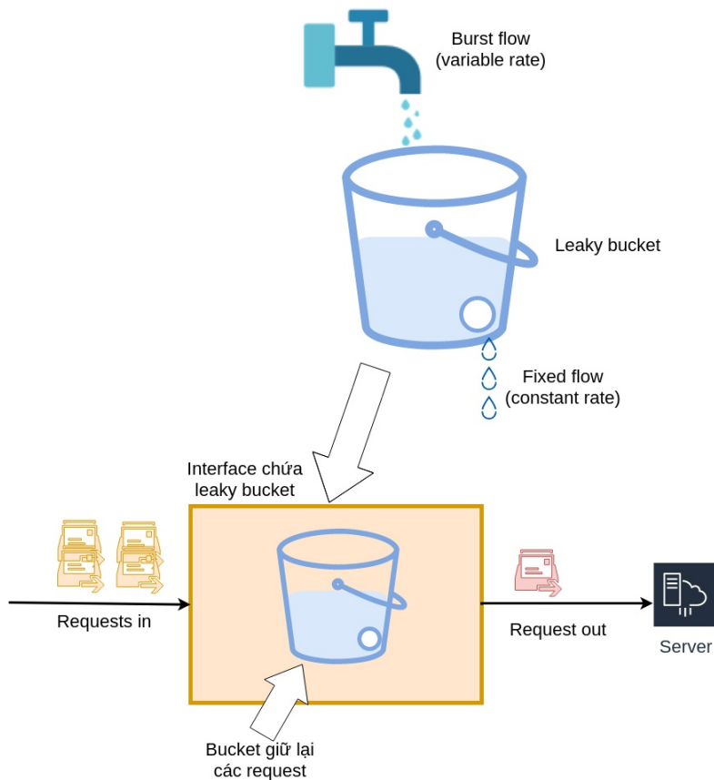
Minh hoạ Leaky bucket
