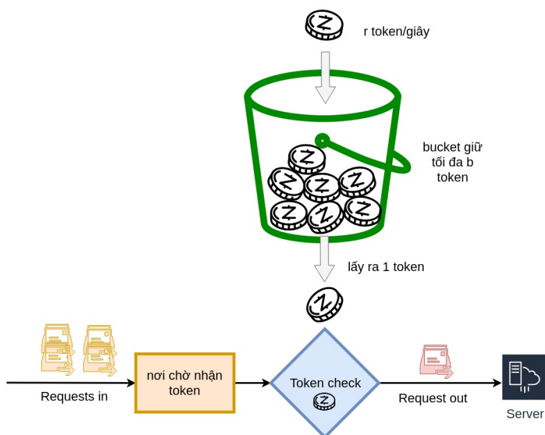
Minh hoạ Token bucket
