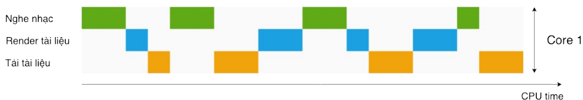
Chia nhỏ tác vụ và xử lý trong mô hình concurrency
