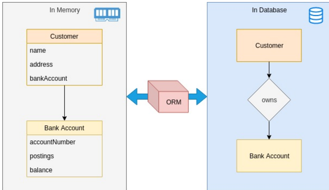
Minh hoạ mapping giữa Database và Struct trong memory
