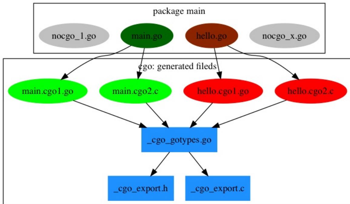
Các file trung gian được CGO tạo ra
