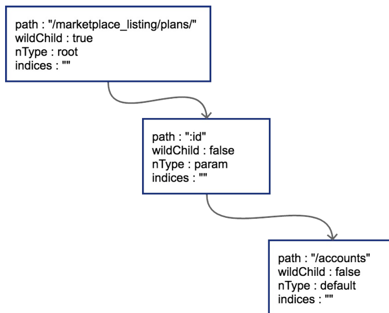
Chèn node thứ hai vào Radix tree
