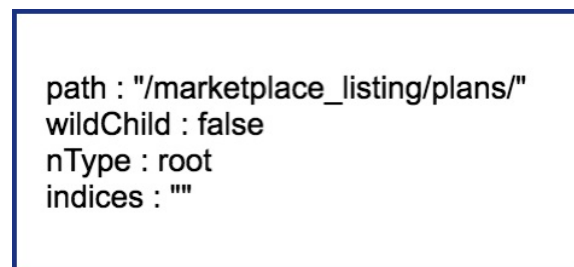
Chèn node đầu tiên vào Radix tree
