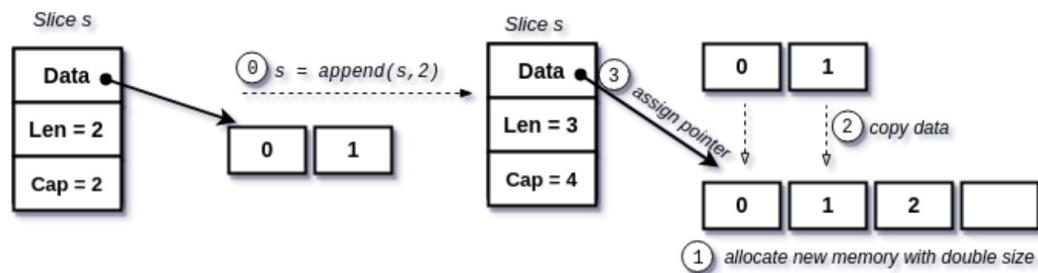
Cấu trúc Slice
