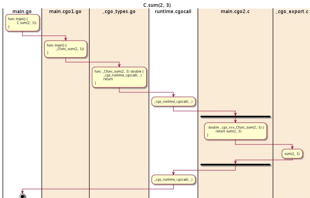
Gọi hàm C
