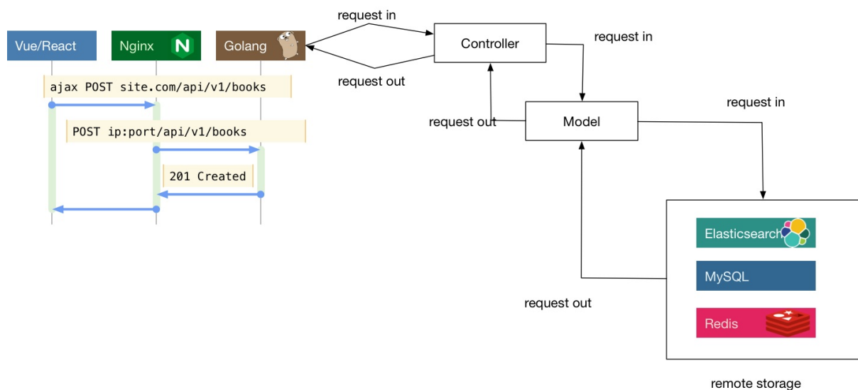
Kiến trúc một dự án web
