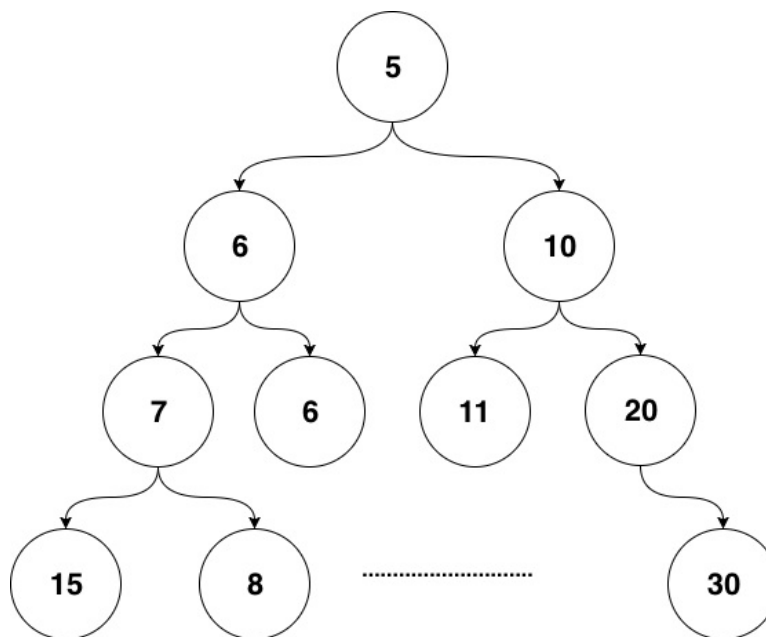
Cấu trúc heap nhị phân
