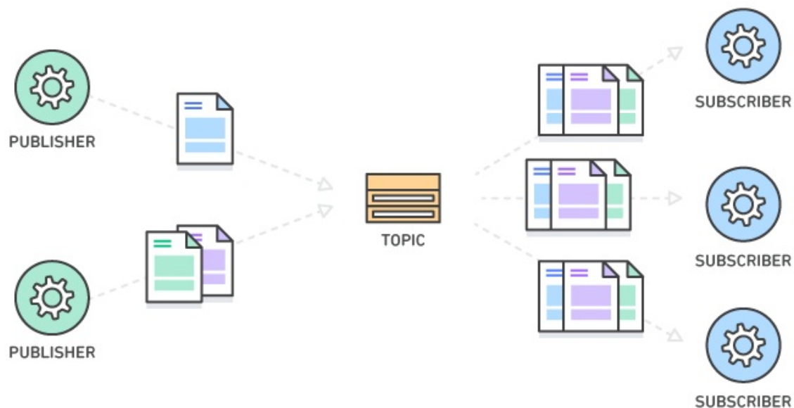
Mô hình Publish - Subscribe
