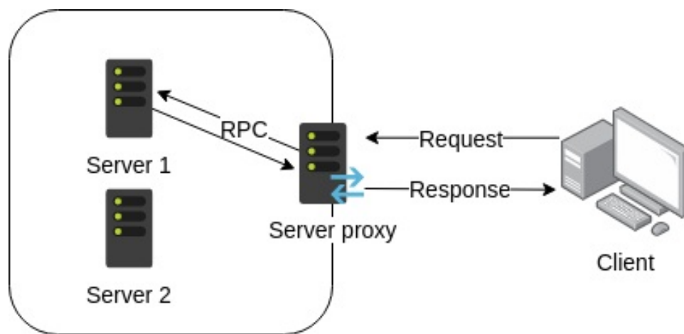
Mô hình dùng reverse proxy
