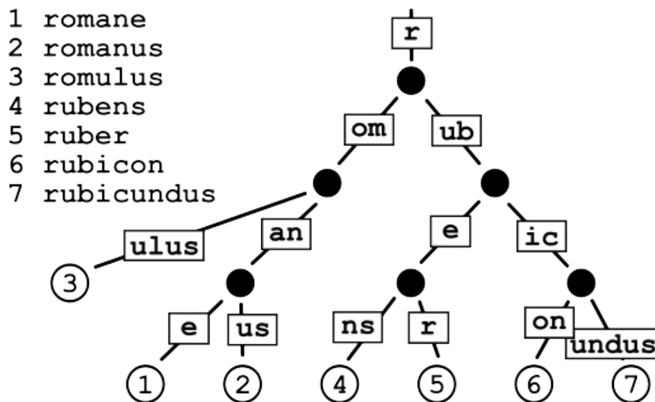
Cây Radix tree
