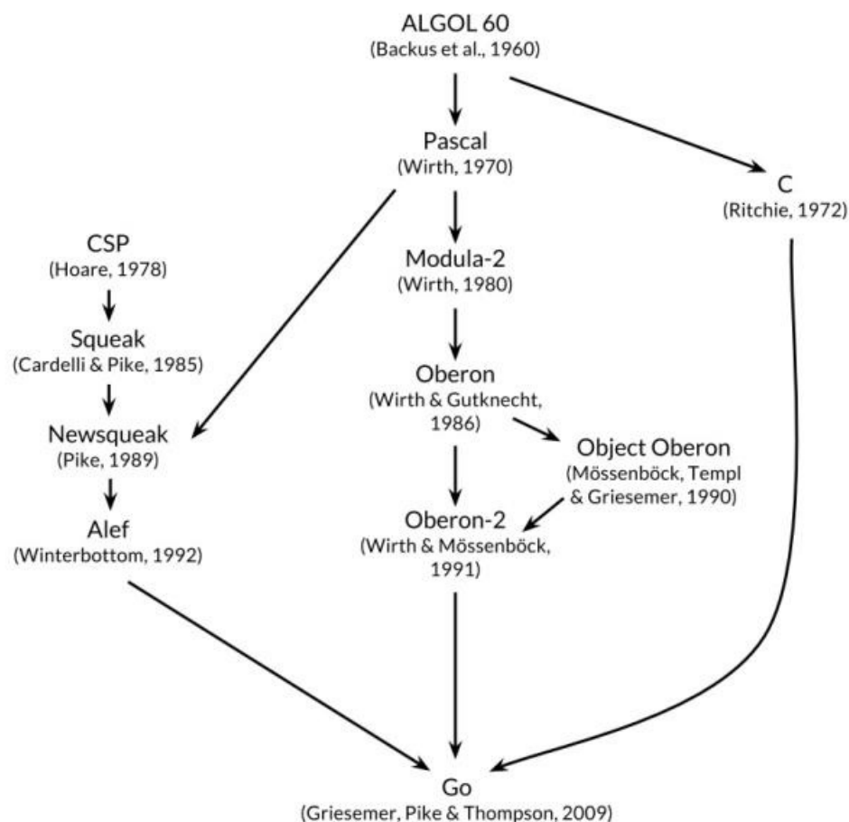
Cây phả hệ của ngôn ngữ Go
