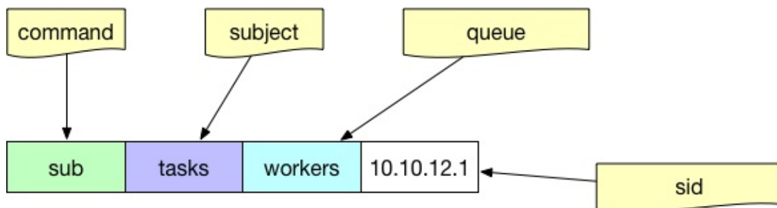
Sub trong giao thức NATS
