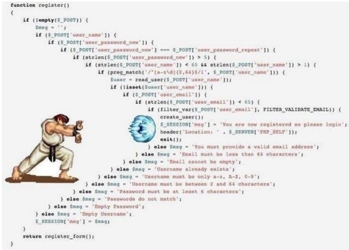
'Hadouken' if-else
