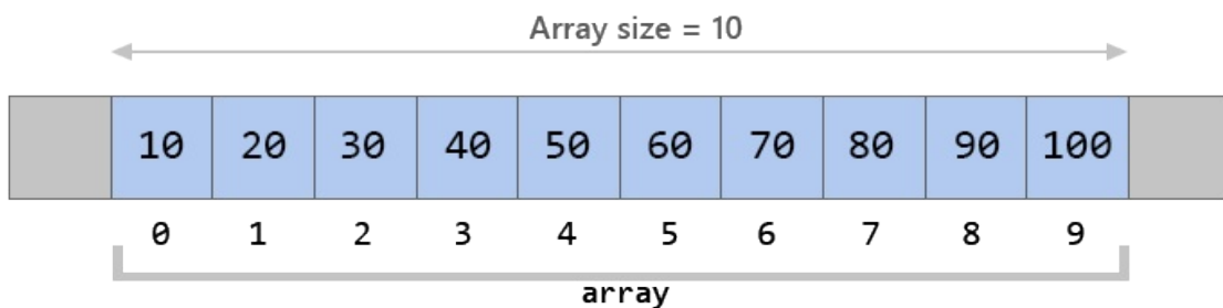
Array
