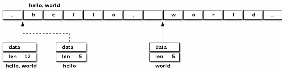
String layout
