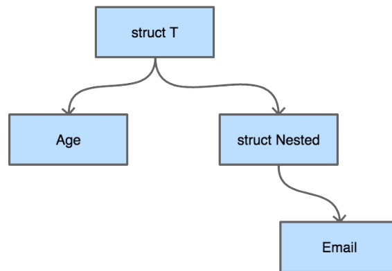
Cây validator
